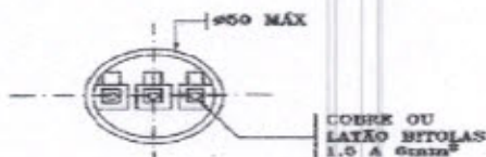
VISTA INFERIOR
